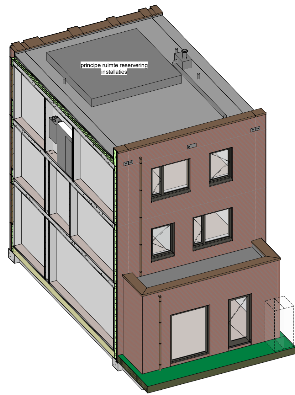
3D-view - Optie 02
