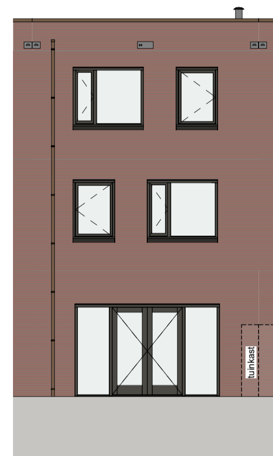
Achtergevel - Optie 01 Schaal: 1 : 100
