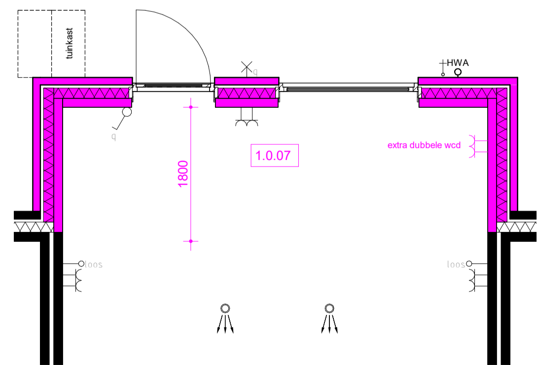
Begane grond - Optie 02 Schaal: 1 : 50 Uitbouw 1800 mm
