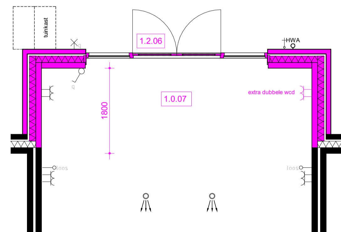
Begane grond - Optie 03 Schaal: 1 : 50 Uitbouw 1800 mm Dubbele deuren met zijlicht
