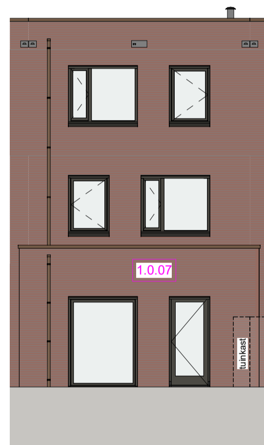
Achtergevel - Optie 02 Schaal: 1 : 100
