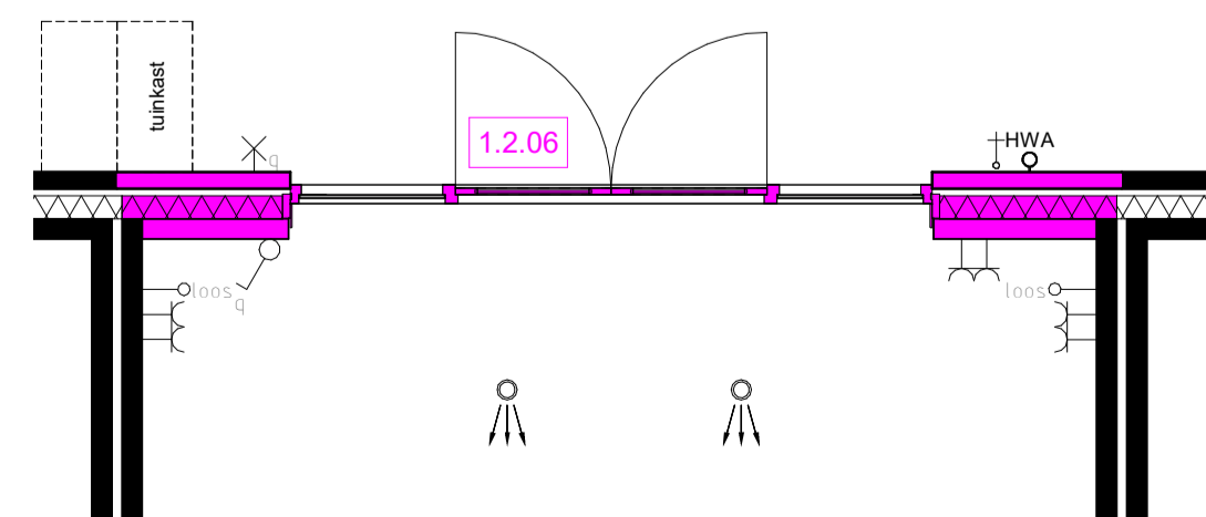
Begane grond - Optie 01 Schaal: 1 : 50 Dubbele deuren met zijlicht
