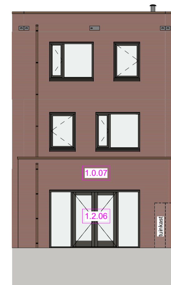
Achtergevel - Optie 03 Schaal: 1 : 100
